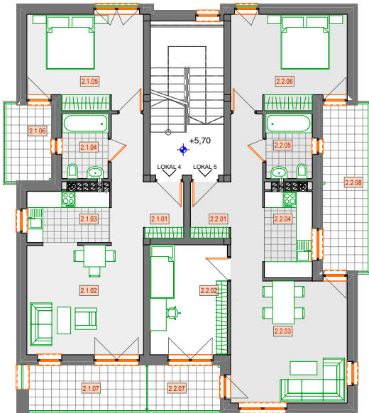
RZUT II PIĘTRA
