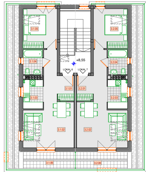
RZUT III PIĘTRA
